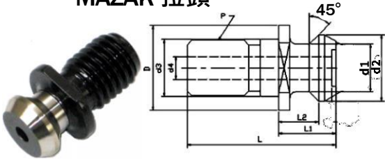
MAZAK 拉頭
